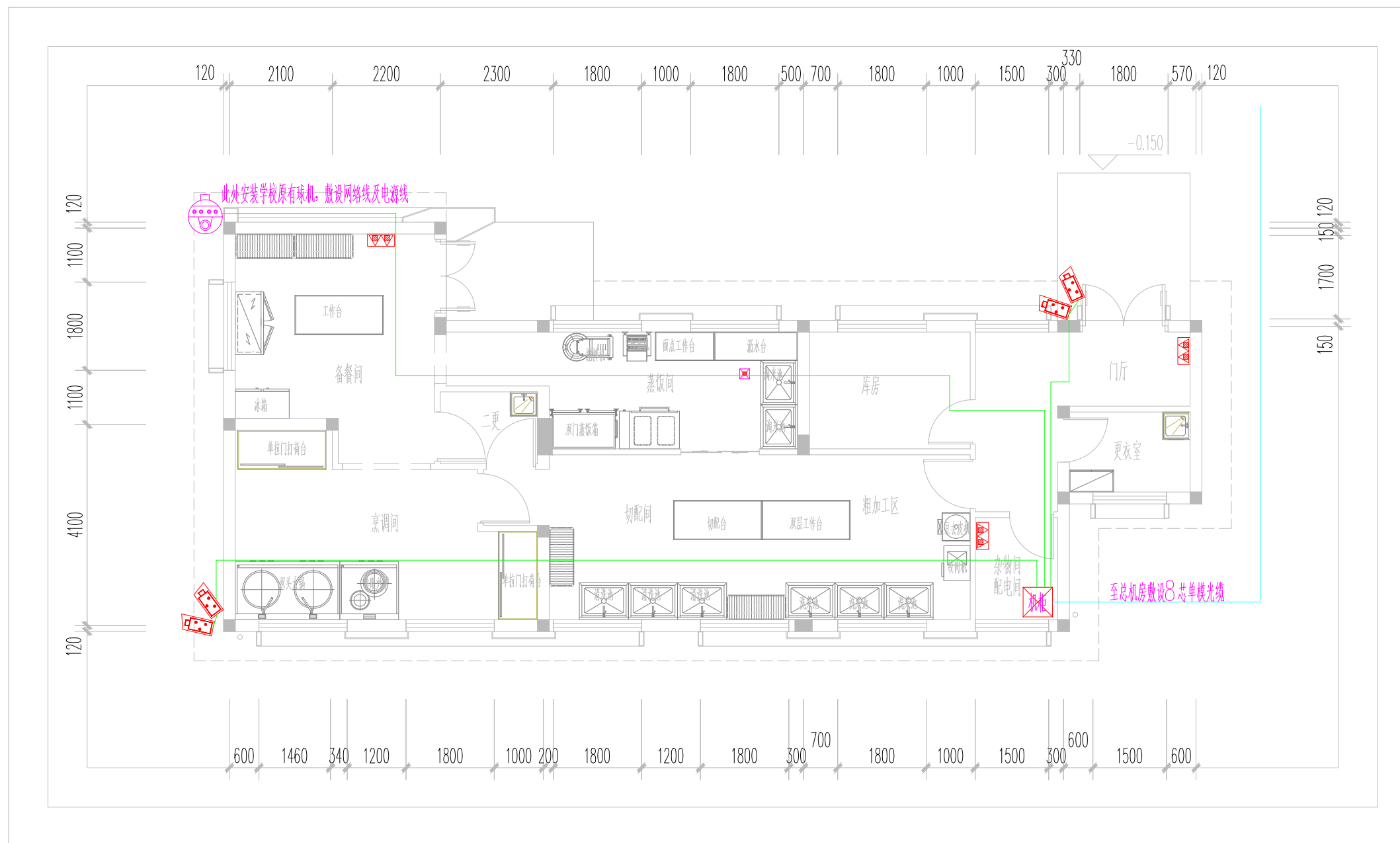
一层平面图 1:100
